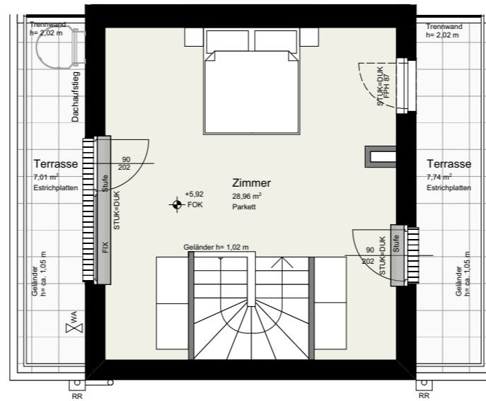
DACHGESCHOSS
