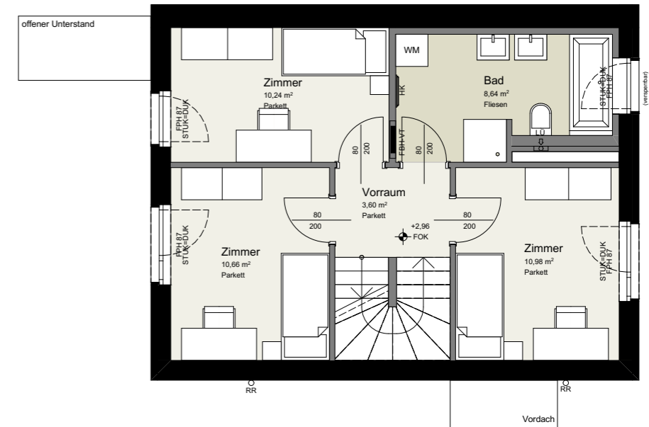
1.OBERGESCHOSS
